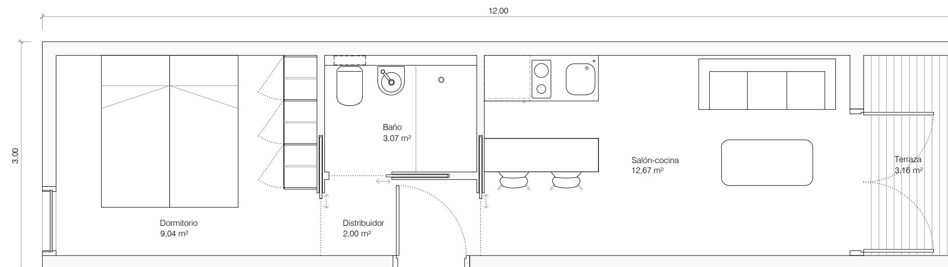
PLANTA
