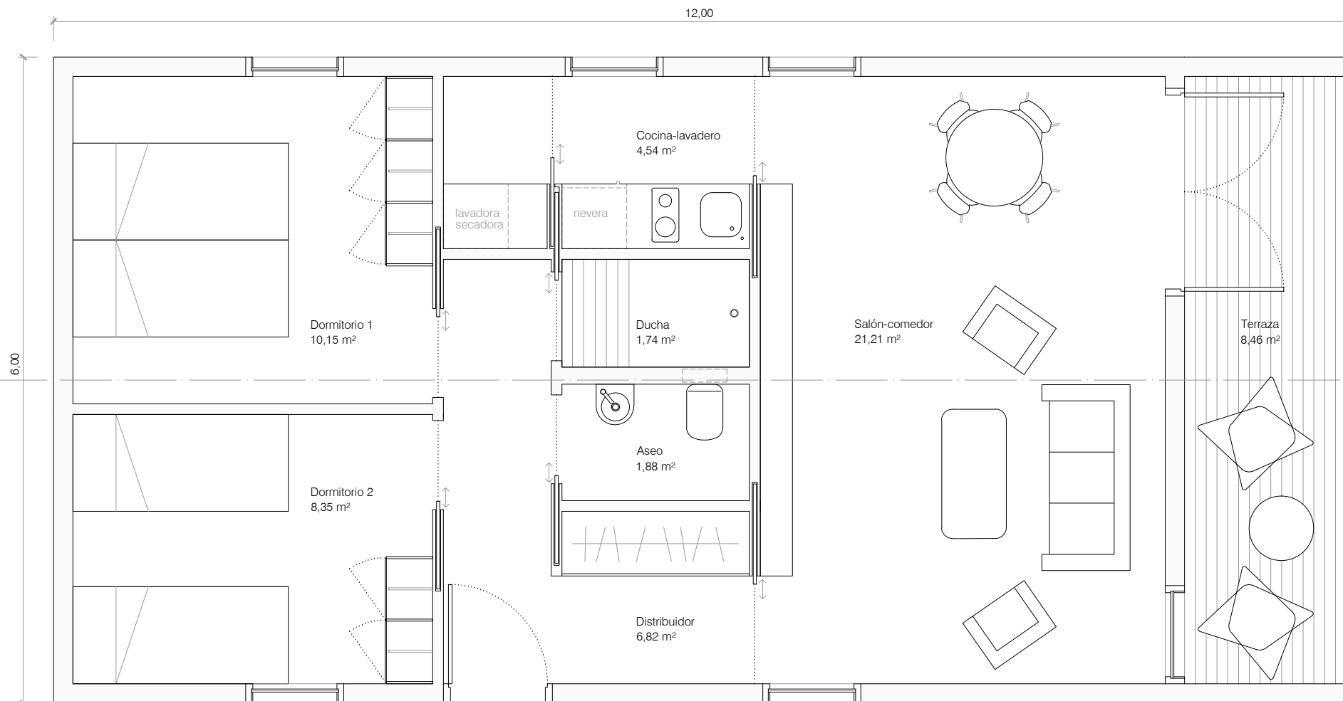
PLANTA
