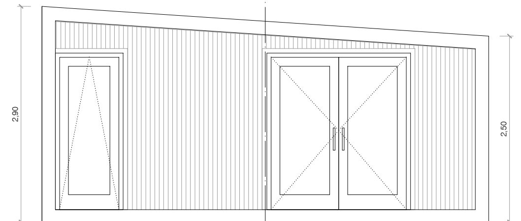
ALZADO TERRAZA
