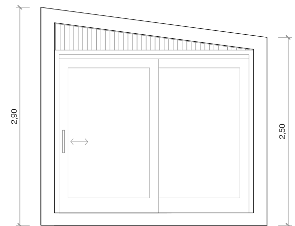
ALZADO TERRAZA
